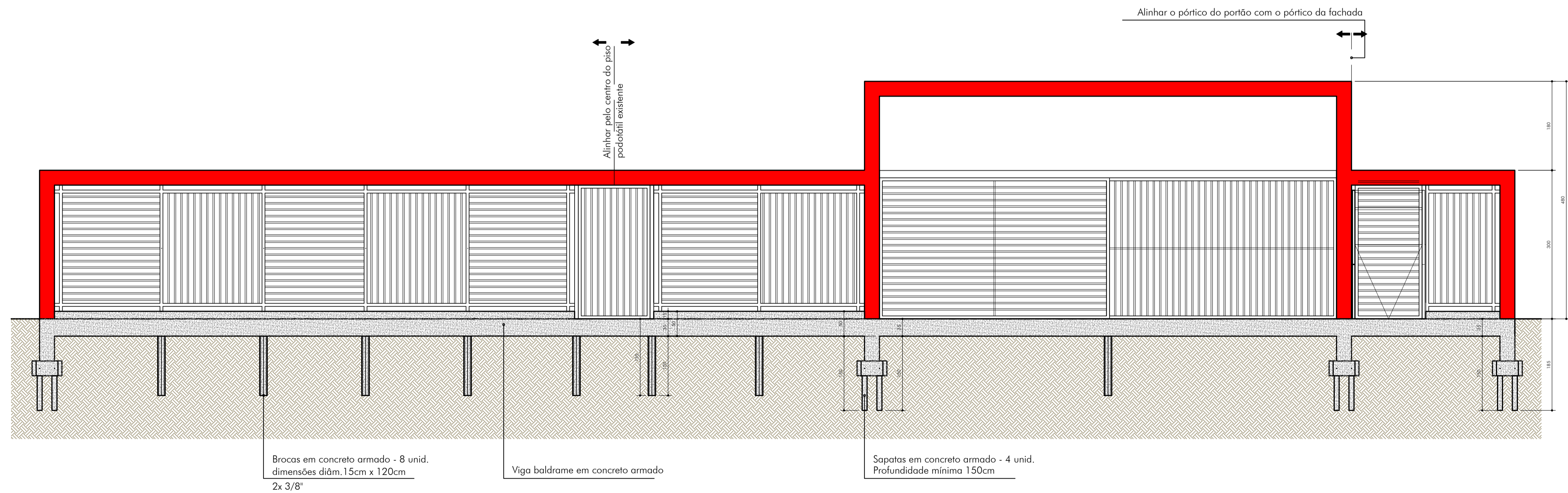
PÓRTICOS, PORTÕES E PASSEIO ESQUEMA ESTRUTURAL - CORTE FONTAL ESCALA 1:50
